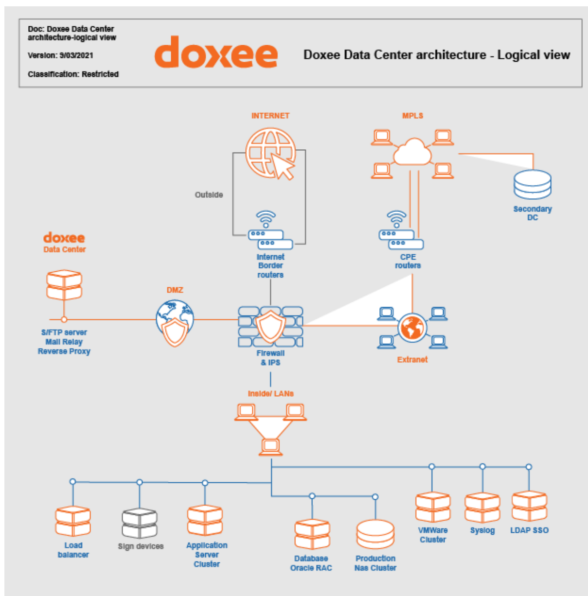
Figura 4. Infrastruttura Hardware
